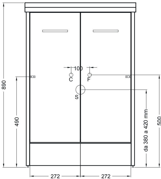
VISTA FRONTALE
